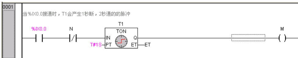
图 3-6-15 程序编写步骤（15）
