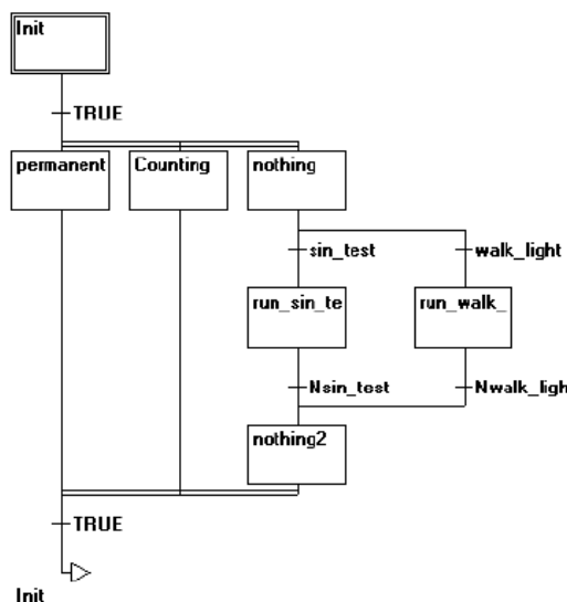
图 9-4-1 顺序功能图语言
