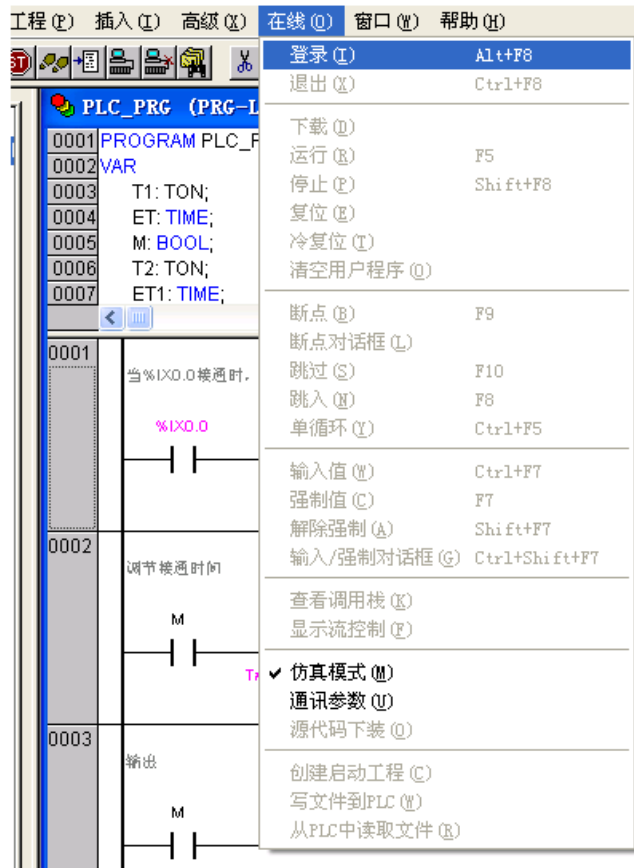
图 3-9-1 仿真模式
