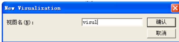
图 11-1-3 视图名称
