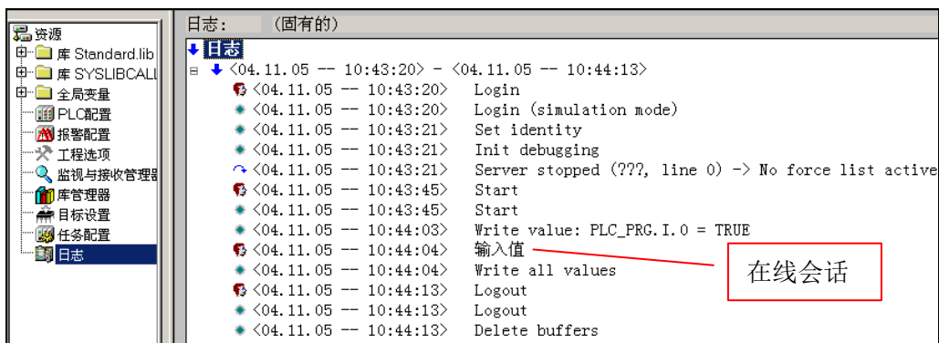
图 7-6-12 日志列表
