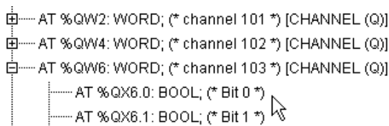
图 10-5-6 输出区地址
