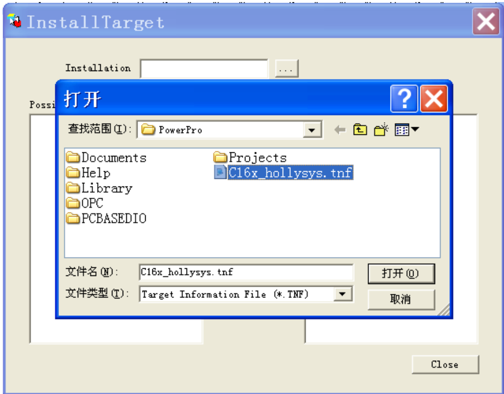
图 1-3-2 安装目标 (2)
