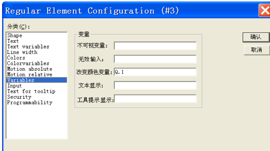
图 11-12-4 变量设置
