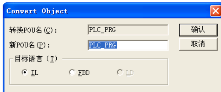
图 2-3-5 语言转换
