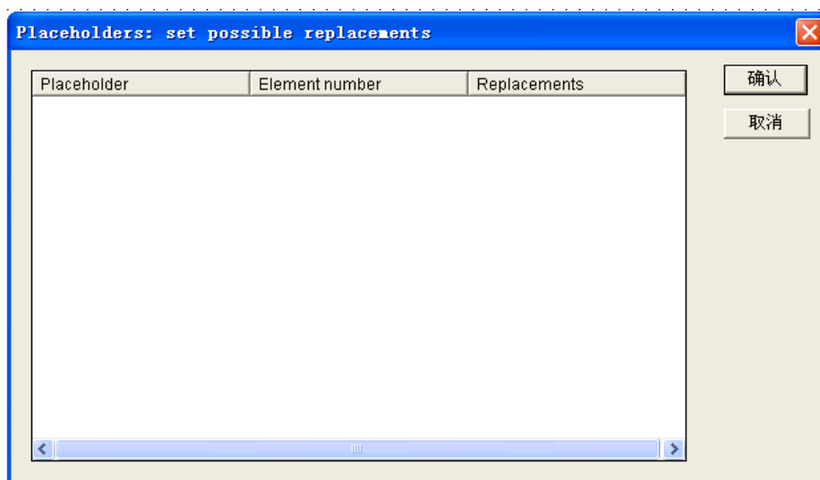
图 11-3-3 占位符列表
