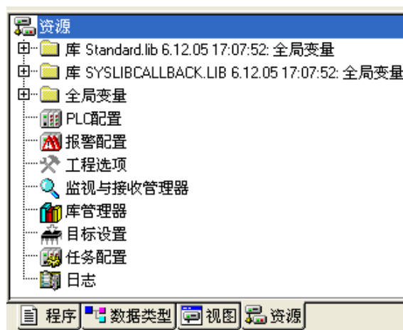
图 2-5-1 对象组织器（1）
