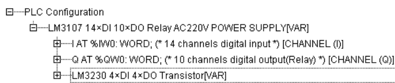
图 7-3-4 添加扩展模块（2）
