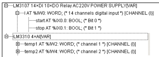
图 7-3-6 I/O 变量定义
