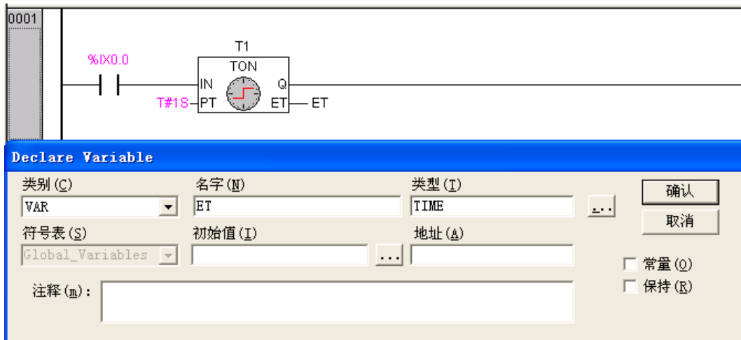
图 3-6-6 程序编写步骤 (6)
