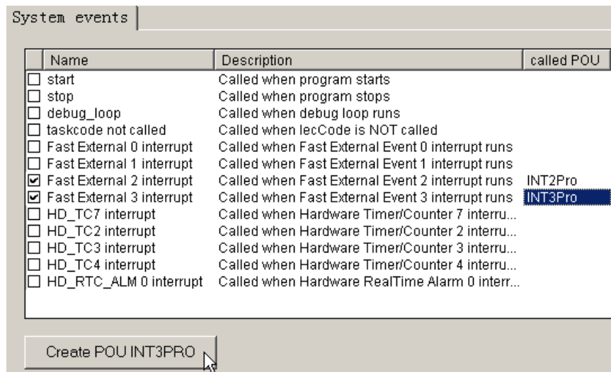
图 10-2-4 创建中断程序
