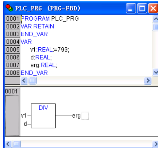
图 5-3-8 函数调用举例（3）
