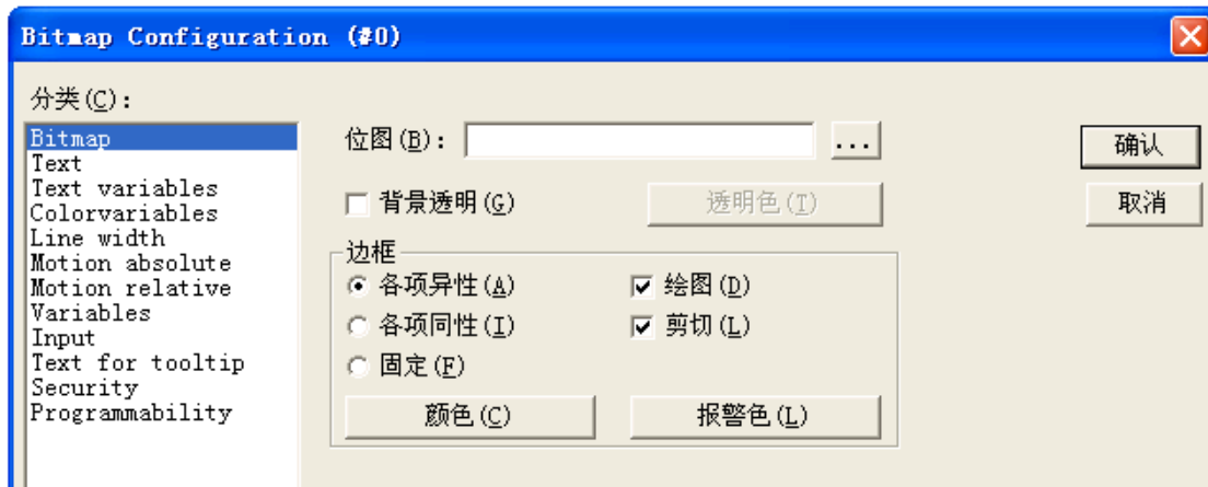
图 11-5-9 位图设置
