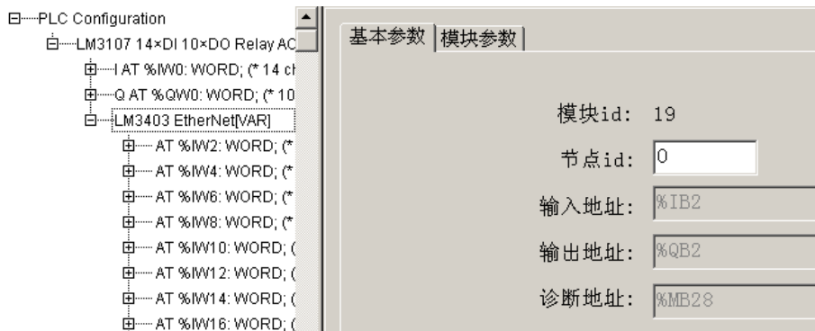
图 10-5-3 EtherNet_TCP 配置表
