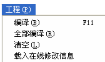
图 8-1-1 工程菜单
