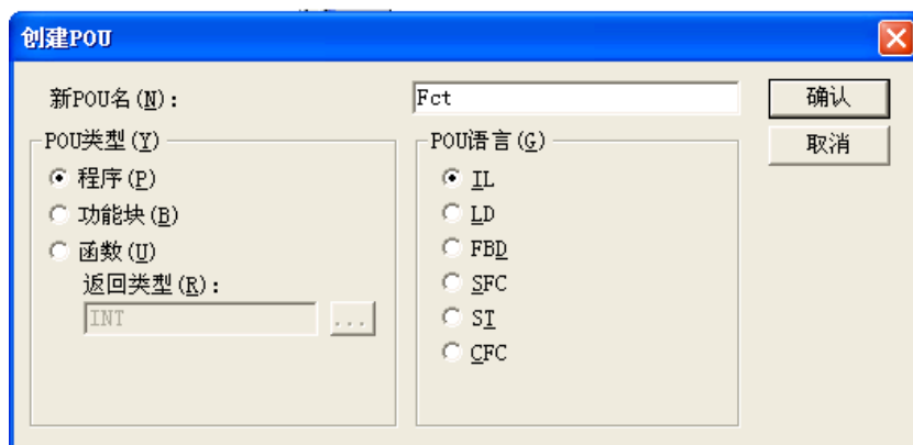
图 5-2-1 创建程序
