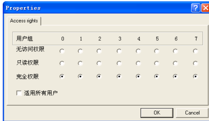
图 2-3-6 属性对话框
