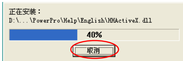
图 1-1-5 安装步骤 (5)
