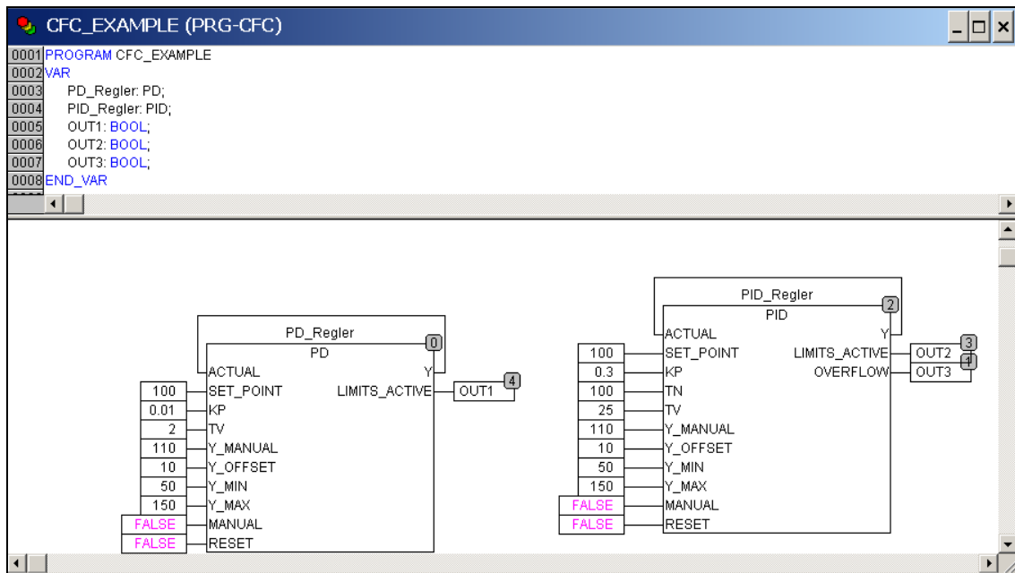
图 9-5-1 CFC 编辑器
