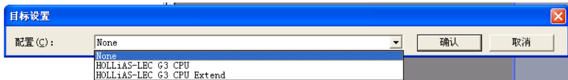
图 7-1-1 选择目标
