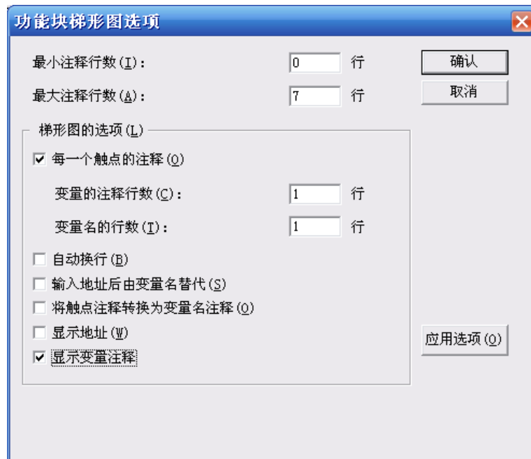
图 7-4-22 梯形图选项
