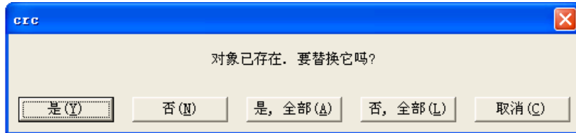
图 7-5-8 覆盖提示
