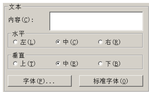
图 11-5-2 文本设置
