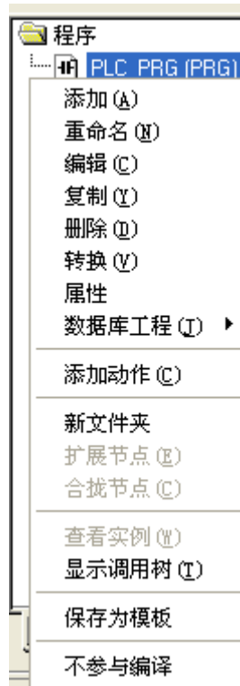
图 2-5-2 程序
