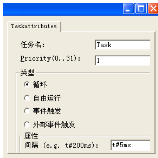
图 6-2-2 任务属性
